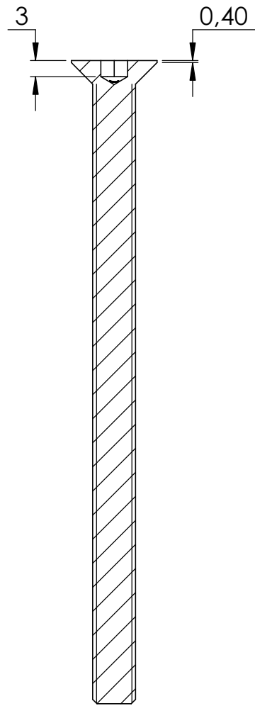
SCHNITT A-A
