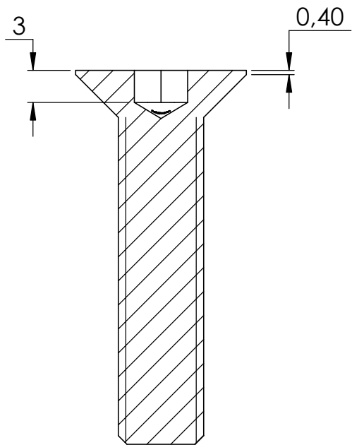
SCHNITT A-A
