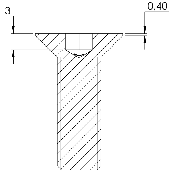
SCHNITT A-A
