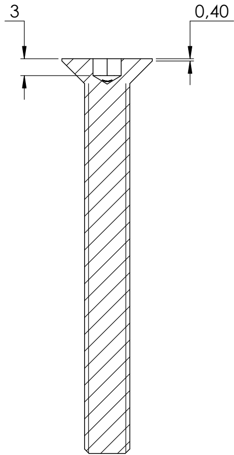
SCHNITT A-A
