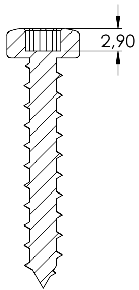
SCHNITT A-A
