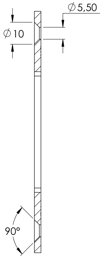
SCHNITT A-A
