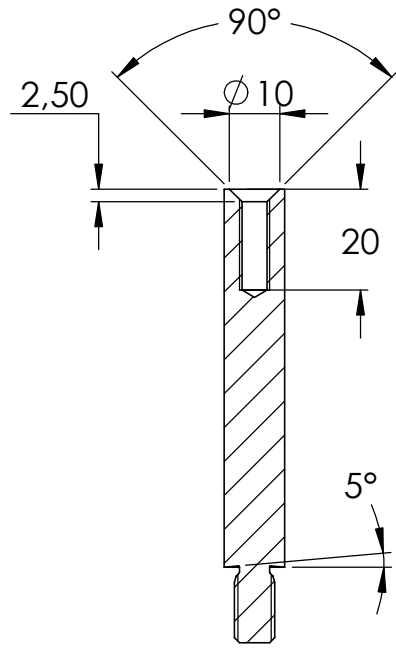
SCHNITT A-A
