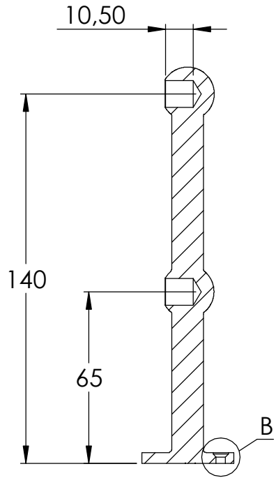
SCHNITT A-A
