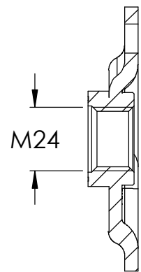
SCHNITT A-A
